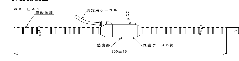
計器概観図
